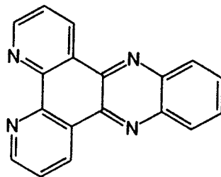
Fig. 1. dppz.
